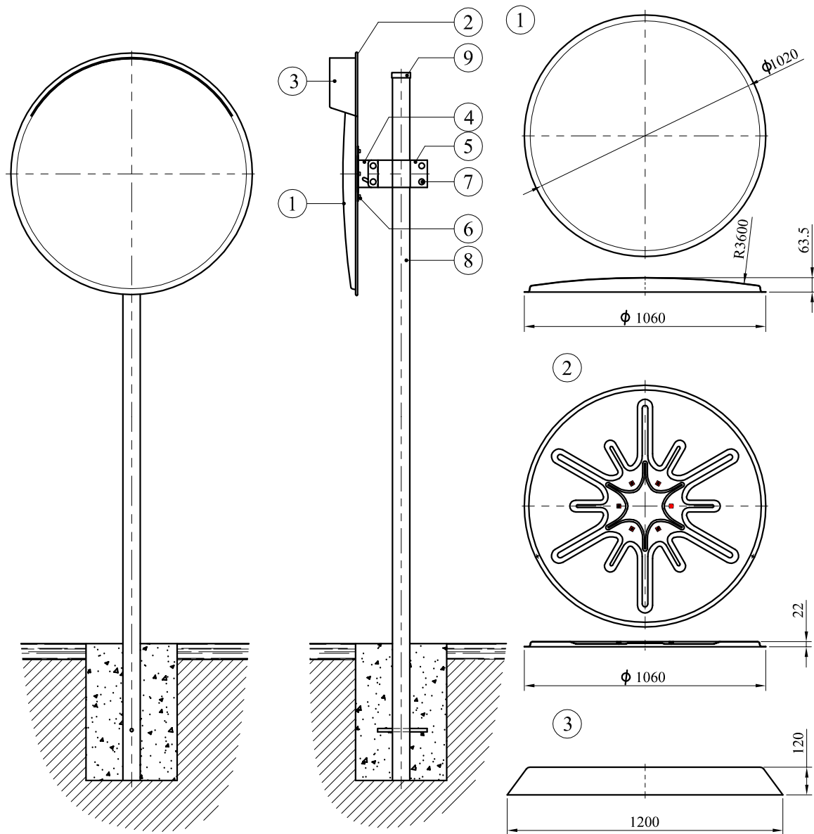
φ100 公分全環保型不銹鋼反射鏡組
