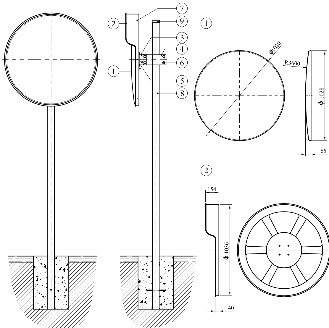
φ100 公分不銹鋼反射鏡組
