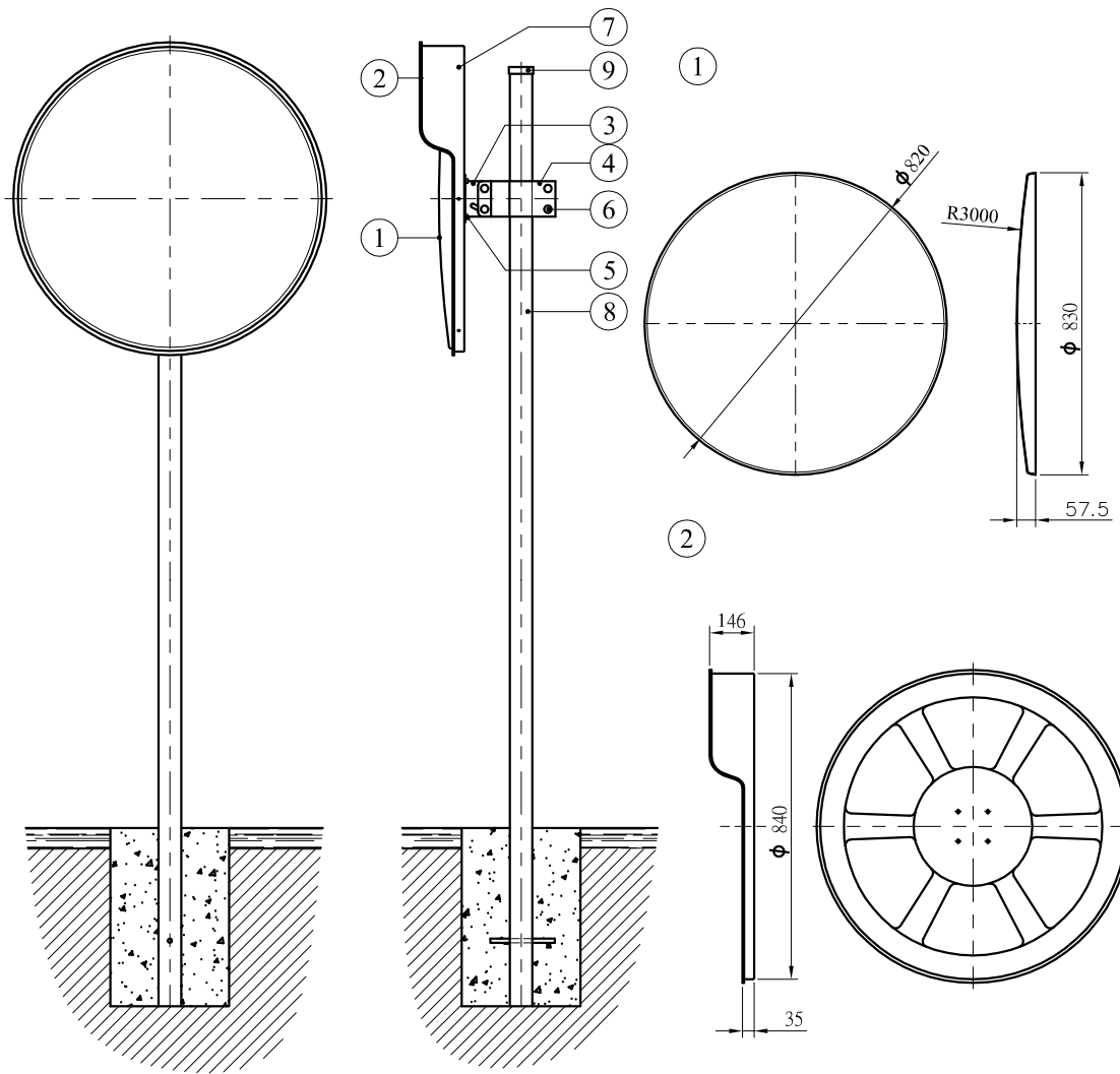
\phi 80 公分不銹鋼反射鏡組
