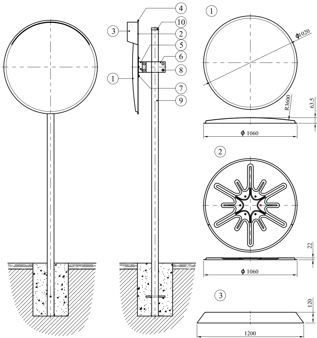
φ100 公分不銹鋼反射鏡組
