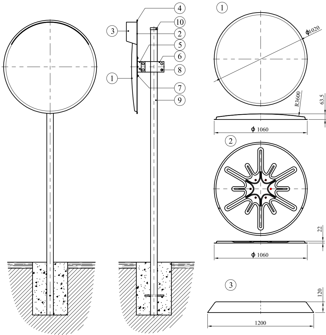
Φ100 公分不銹鋼反射鏡組
