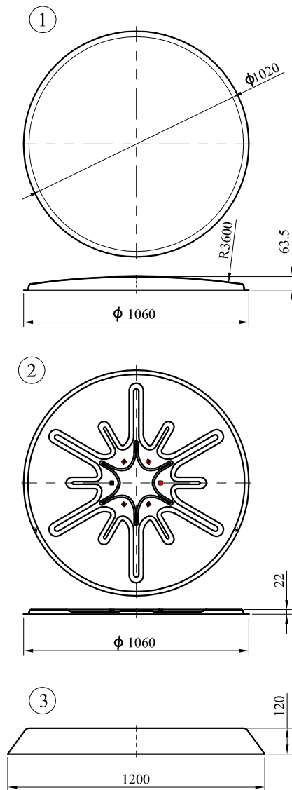
φ100 公分全環保型不銹鋼反射鏡組
