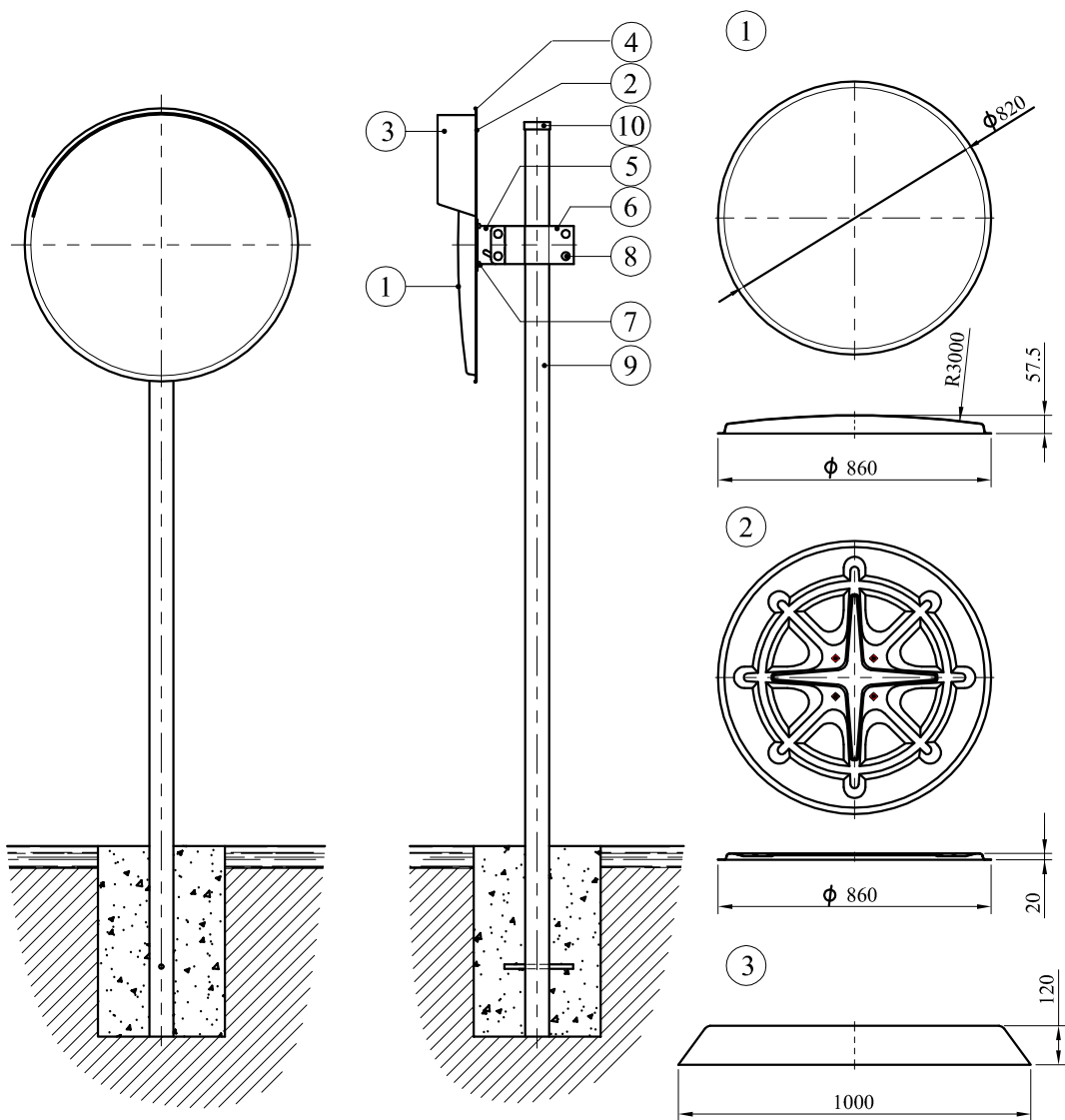
φ80公分不銹鋼反射鏡組
