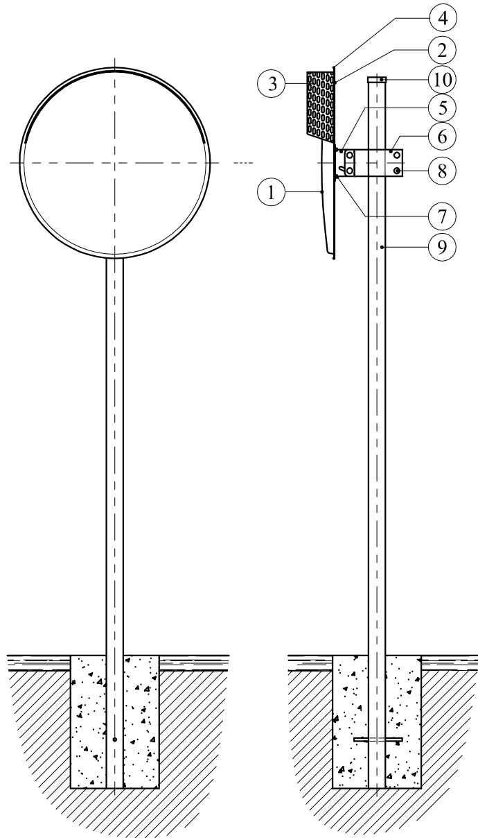
\phi 80 公分不銹鋼反射鏡組
